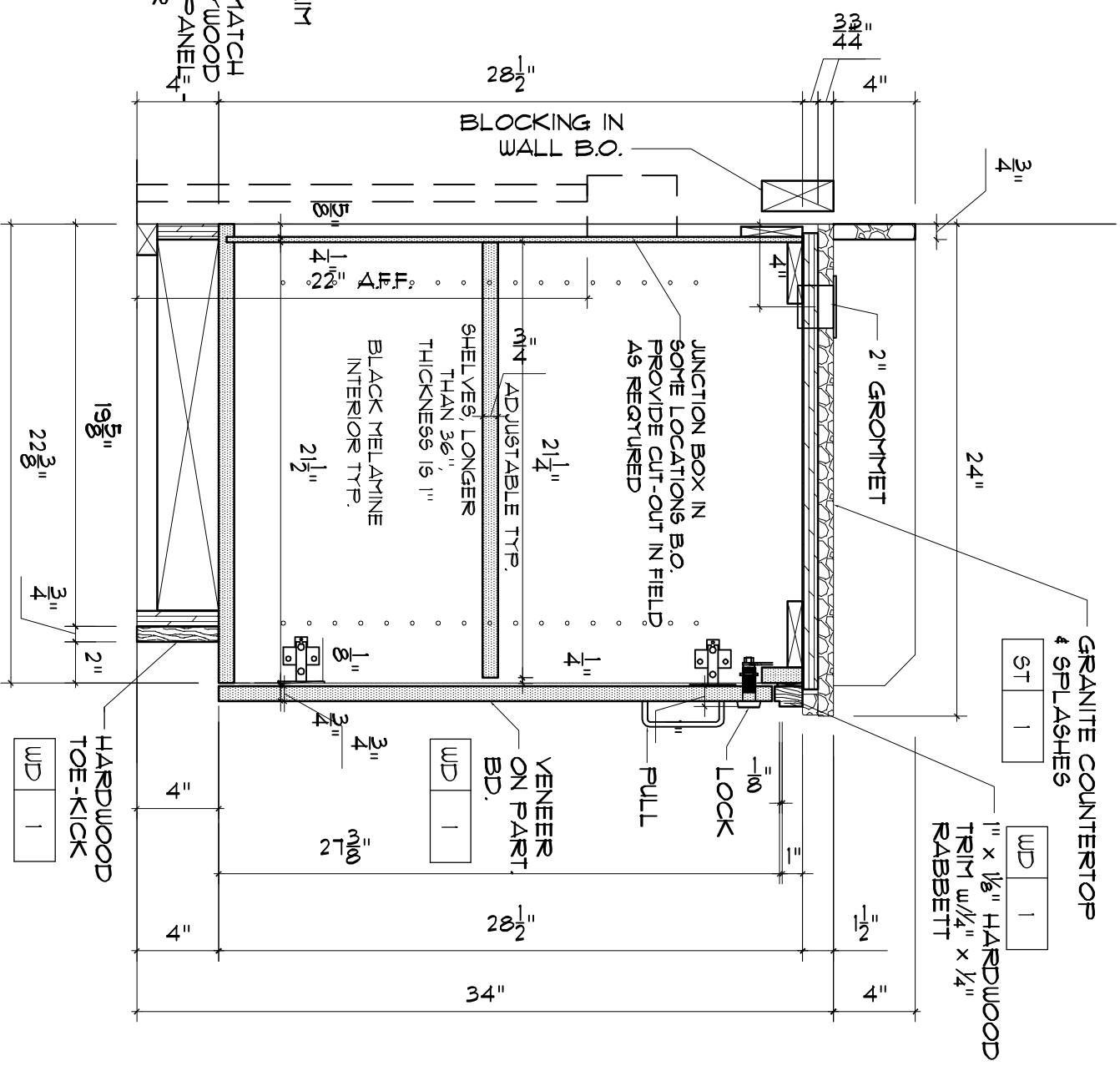
SECTION 3 SCALE: 1-1/2"=1'-0"
